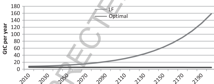
f0080 Fig. 15 Fossil fuel use: optimum vs laissez faire.
